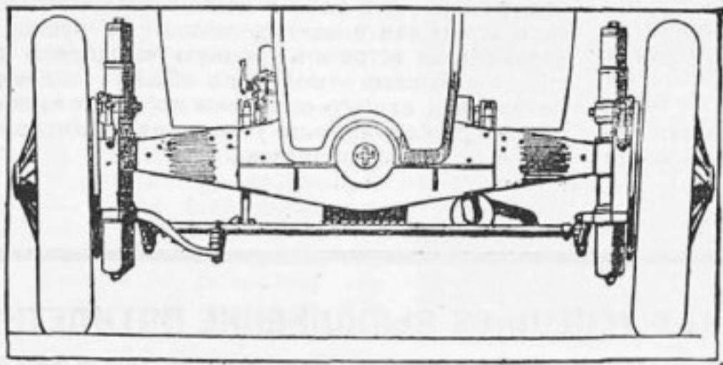
Рис. 2. Общий вид установленных на машине амортизаторов
