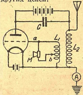
Рис. 2. Схема телефонного передатчика с последовательным питанием
